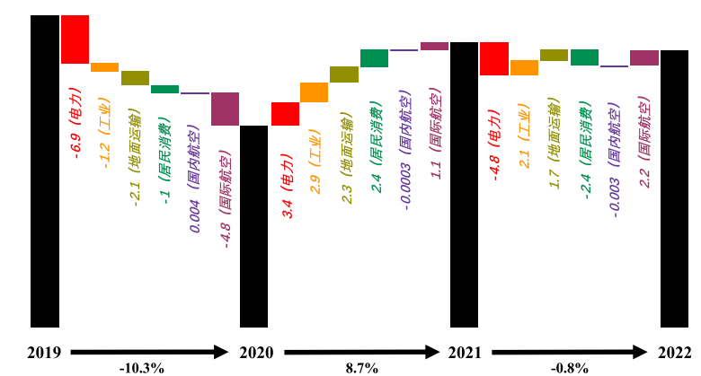
荷兰各部门二氧化碳排放变化
