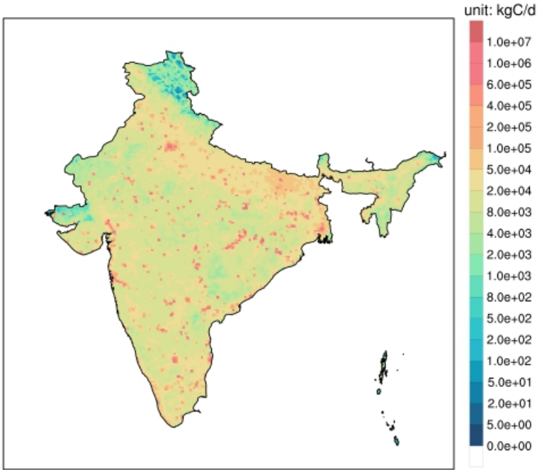
图3-90 2020年印度日均碳排放地图
