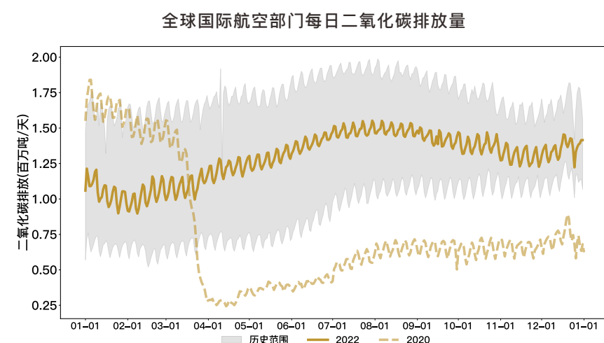
图2-14 2019年1月1日至2022年12月31日国际航空部门二氧化碳排放日度变化情况
