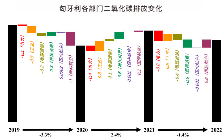
图3-75 2019-2022年匈牙利二氧化碳排放总量（黑色柱子）与各部门排放变化情况（彩色柱子）
