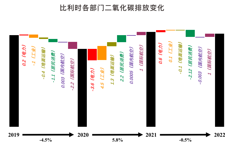
图3-39 2019-2022年比利时二氧化碳排放总量（黑色柱子）与各部门排放变化情况（彩色柱子）
