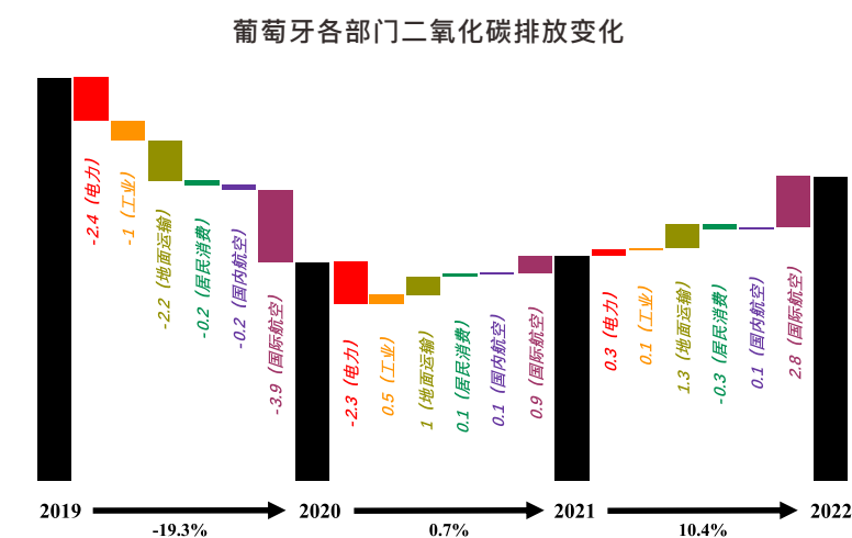
图3-63 2019-2022年葡萄牙二氧化碳排放总量（黑色柱子）与各部门排放变化情况（彩色柱子）
