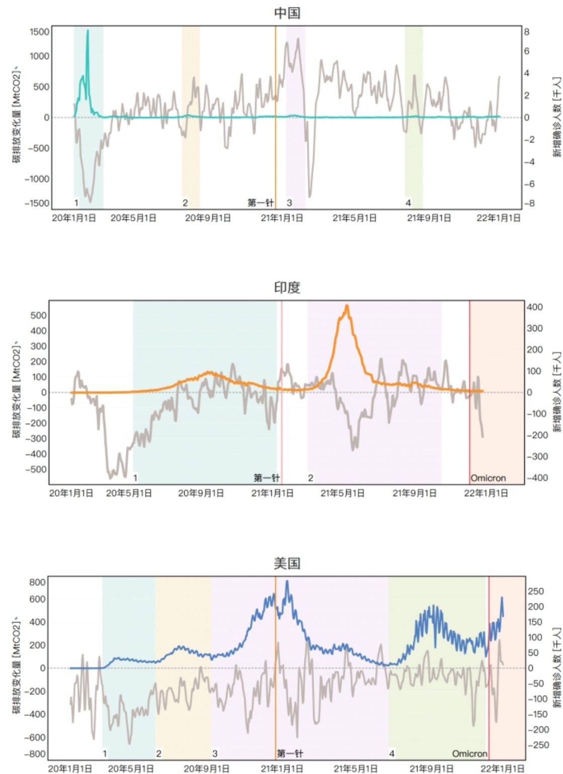
图4-3 全球实时碳数据展示中国、印度、美国天尺度碳排放变量
