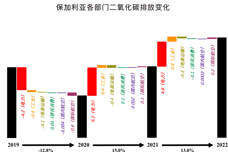
图3-37 2019-2022年保加利亚二氧化碳排放总量(黑色柱子)与各部门排放变化情况(彩色柱子)
