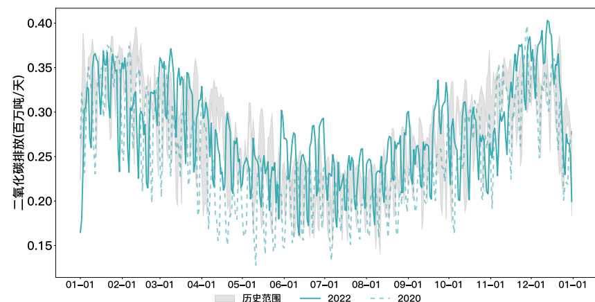
图3-48 2019年1月1日至2022年12月31日捷克每日二氧化碳排放量
