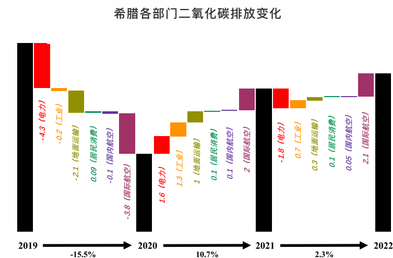
图3-73 2019-2022年希腊二氧化碳排放总量（黑色柱子）与各部门排放变化情况（彩色柱子）
