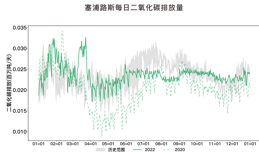
图3-66 2019年1月1日至2022年12月31日塞浦路斯每日二氧化碳排放量
