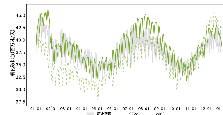
图2-4 2019年1月1日至2022年12月31日电力部门二氧化碳排放日度变化情况
