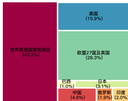
图2-11 2020年世界各国居民消费部门二氧化碳排放在全球居民消费部门二氧化碳总排放中占比
