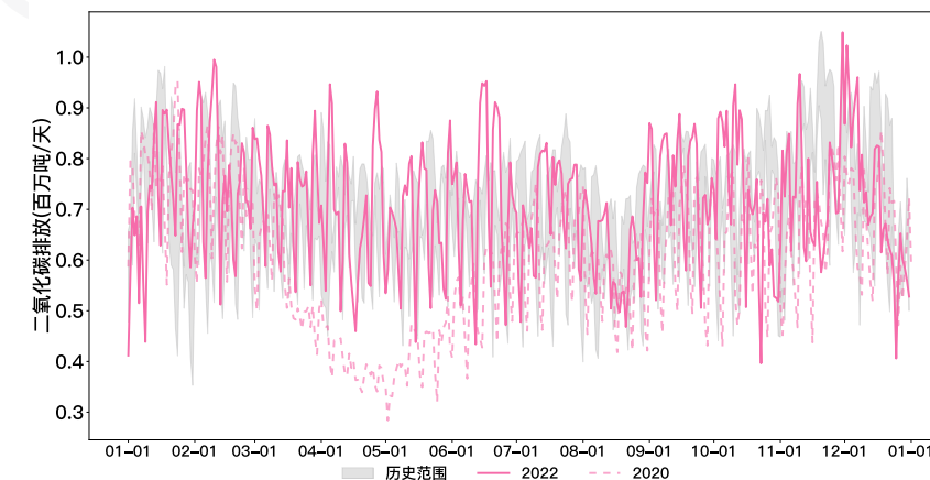
图3-27 2019年1月1日至2022年12月31日西班牙二氧化碳排放日度变化情况
