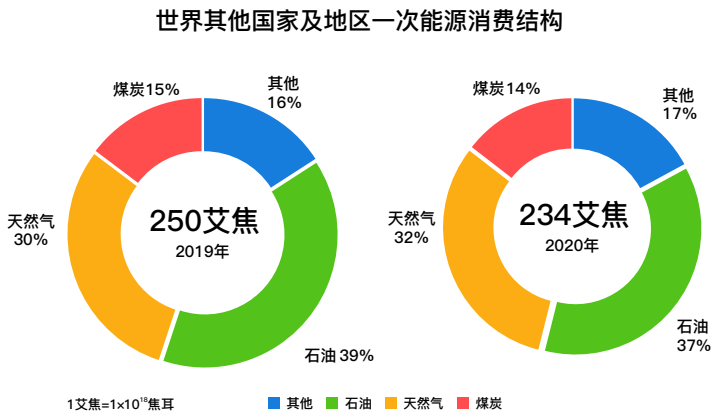
图3-95 世界其他国家和地区一次能源消费结构
