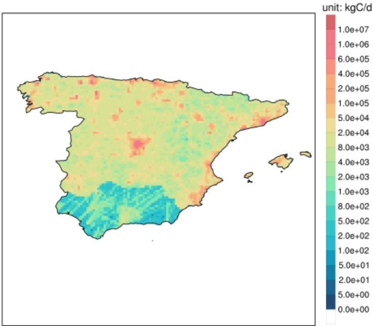
图3-29 2020年西班牙日均碳排放地图
