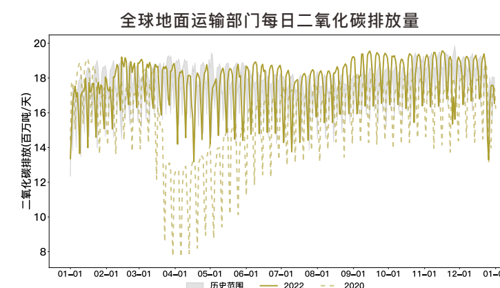
图2-8 2019年1月1日至2022年12月31日地面运输部门二氧化碳排放日度变化情况
