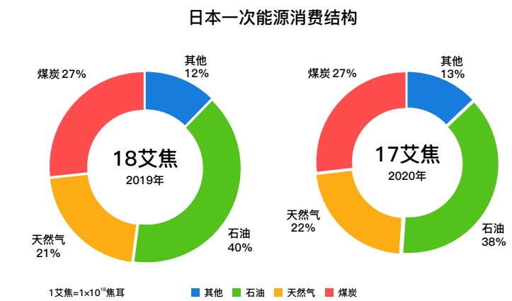
图3-76 日本一次能源消费结构
