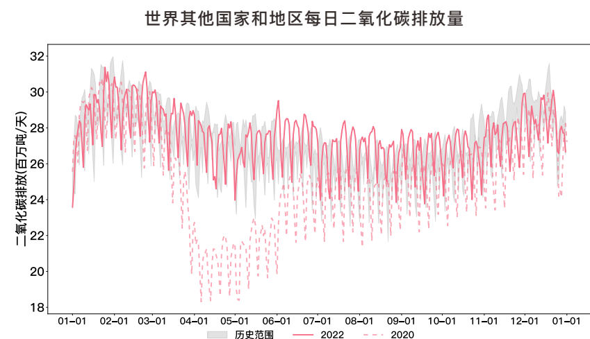
图3-96 2019年1月1日至2022年12月31日世界其他国家及地区二氧化碳排放日度变化情况
