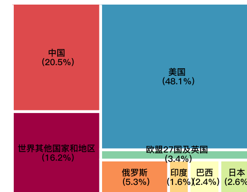
图2-13 2020年世界各国国内航空部门二氧化碳排放在全球国内航空部门二氧化碳总排放中占比
