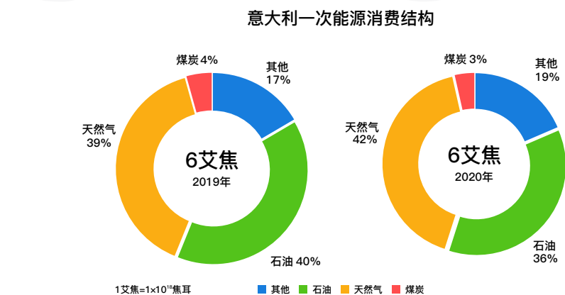
图3-22 意大利一次能源消费结构
