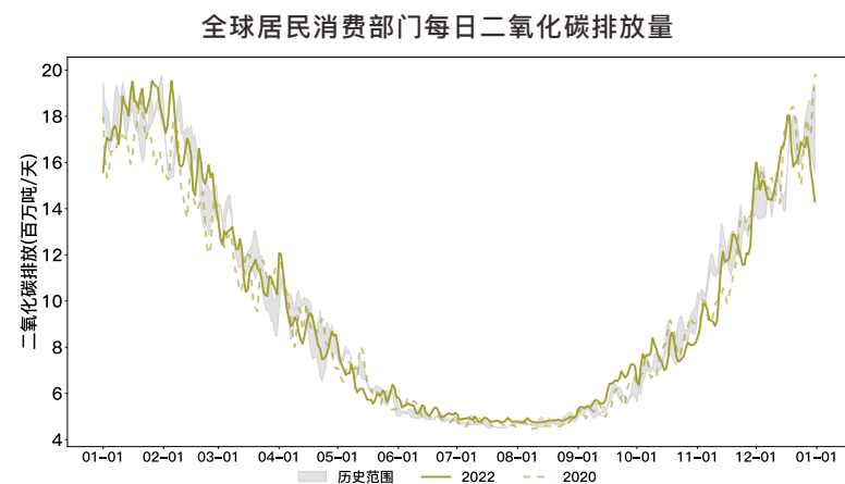
图2-10 2019年1月1日至2022年12月31日居民消费部门二氧化碳排放日度变化情况
