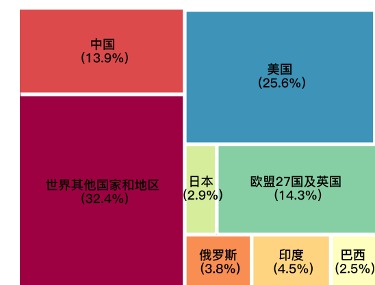
图2-9 2020年世界各国地面运输部门二氧化碳排放在全球地面运输部门二氧化碳总排放中占比
