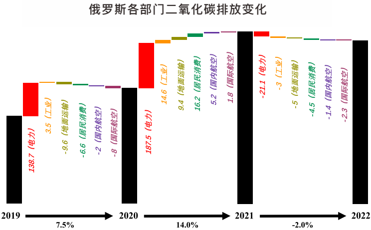
图3-82 2019-2022年 俄罗斯二氧化碳排放总量（黑色柱子）与各部门排放变化情况（彩色柱子）
