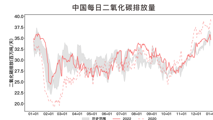
图3-85 2019年1月1日至2022年12月31日中国二氧化碳排放日度变化情况
