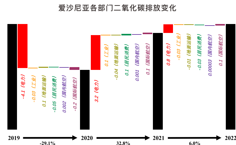
图3-35 2019-2022年爱沙尼亚二氧化碳排放总量（黑色柱子）与各部门排放变化情况（彩色柱子）
