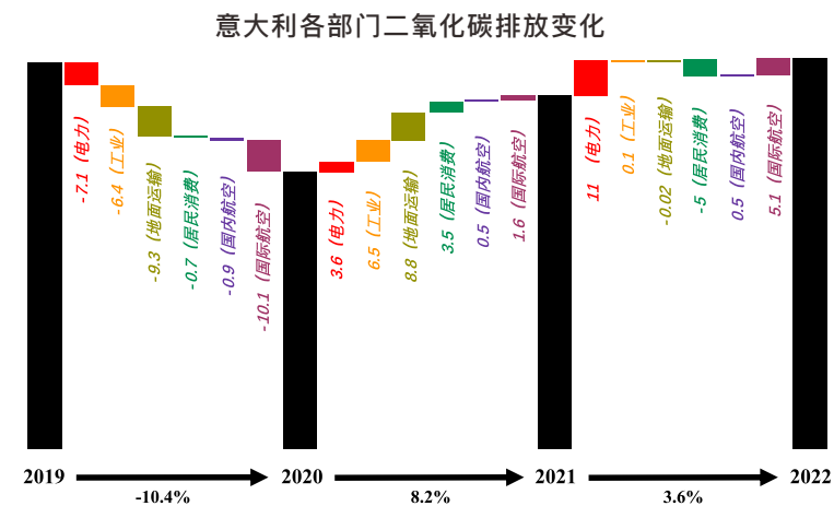
图3-24 2019-2022年意大利二氧化碳排放总量（黑色柱子）与各部门排放变化情况（彩色柱子）
