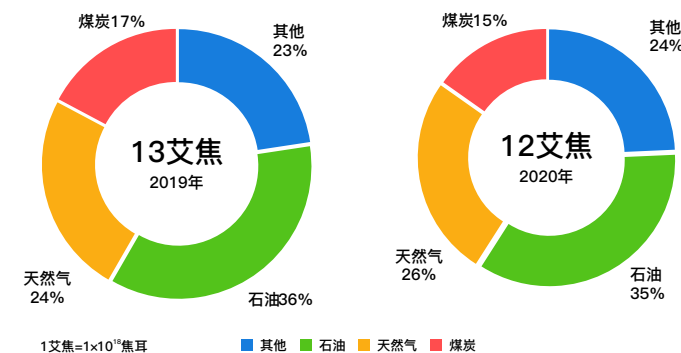
图3-14 一次能源消费结构
