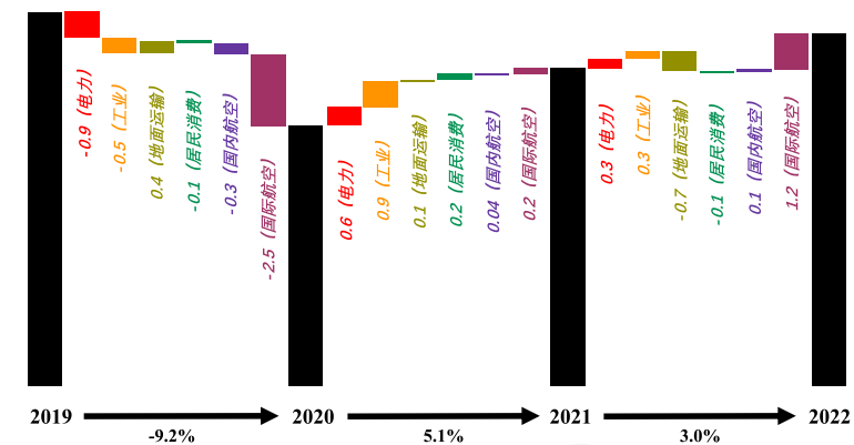
图3-65 2019–2022年瑞典二氧化碳排放总量（黑色柱子）与各部门排放变化情况（彩色柱子）
