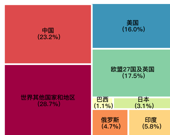
图2-15 2020年世界各国国际航空部门二氧化碳排放在全球国际航空部门二氧化碳总排放中占比
