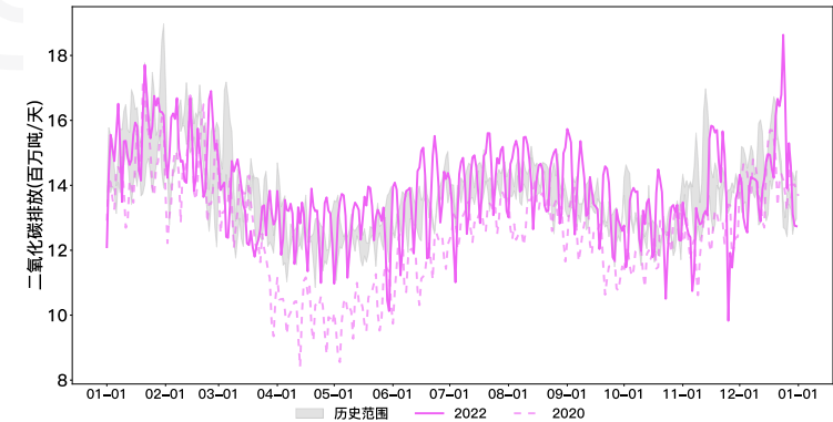
图3-3 2019年1月1日至2022年12月31日美国二氧化碳排放日度变化情况
