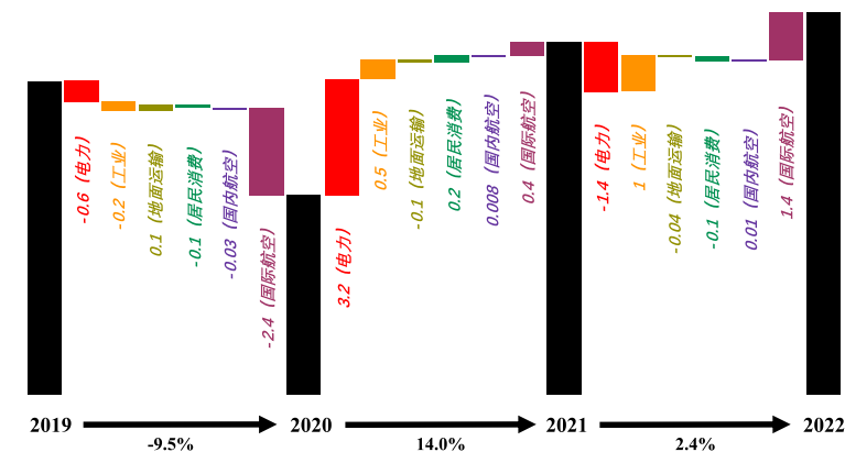
图3-43 2019–2022年丹麦二氧化碳排放总量（黑色柱子）与各部门排放变化情况（彩色柱子）
