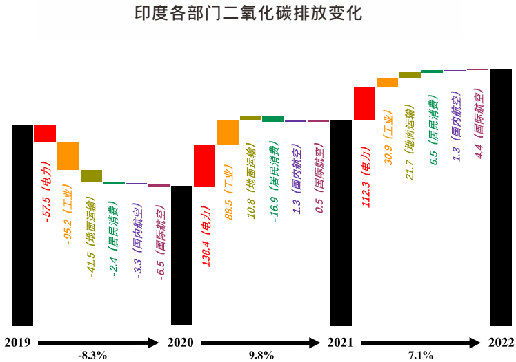
图3-89 2019-2022年 印度二氧化碳排放总量（黑色柱子）与各部门排放变化情况（彩色柱子）
