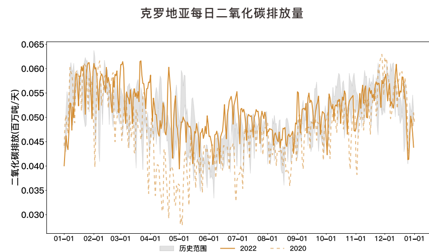
图3-50 2019年1月1日至2022年12月31日克罗地亚每日二氧化碳排放量
