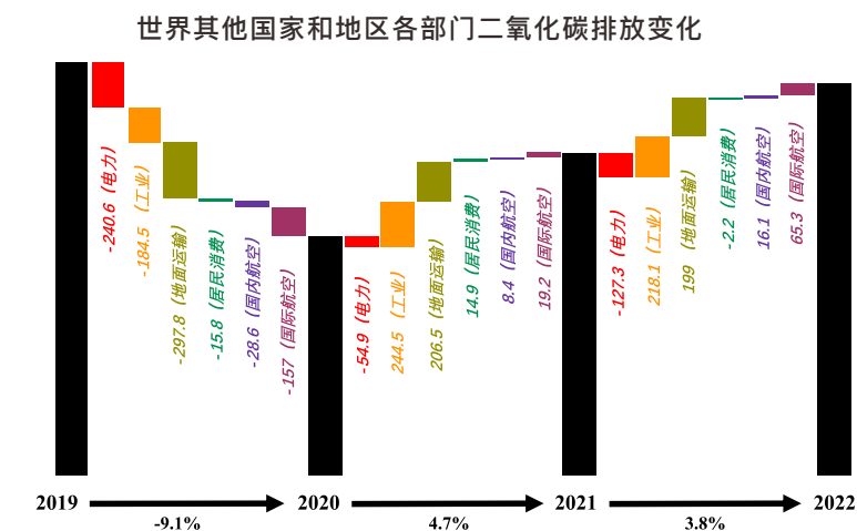
图3-97 2019–2022年世界其他国家及地区二氧化碳排放总量（黑色柱子）与各部门排放变化情况（彩色柱子）
