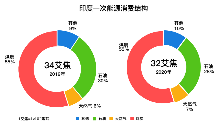
图3-87 印度一次能源消费结构
