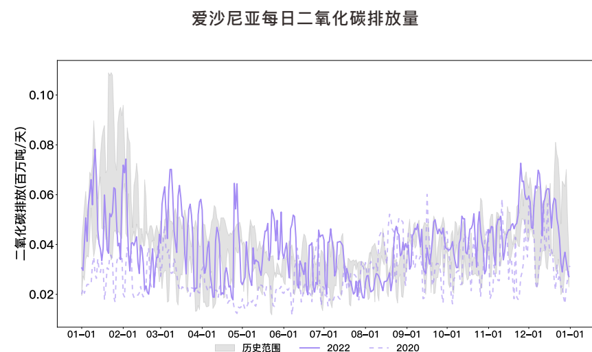
图3-34 2019年1月1日至2022年12月31日爱沙尼亚每日二氧化碳排放量
