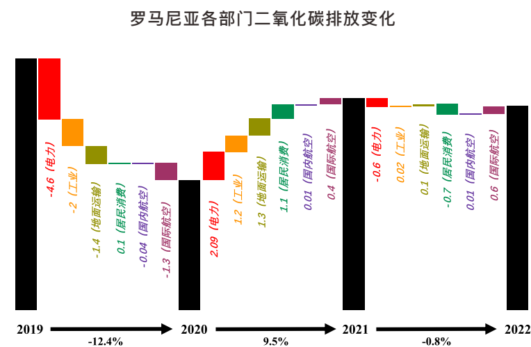
图3-59 2019-2022年罗马尼亚二氧化碳排放总量(黑色柱子)与各部门排放变化情况(彩色柱子)
