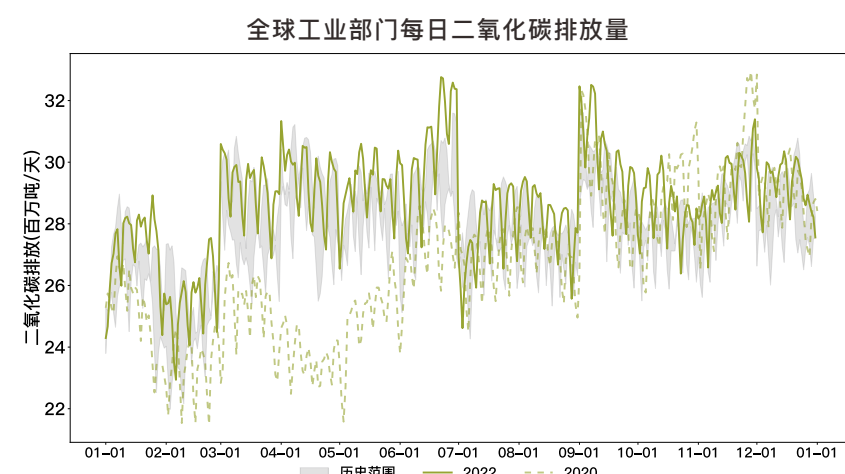
图2-6 2019年1月1日至2022年12月31日工业部门二氧化碳排放日度变化情况
