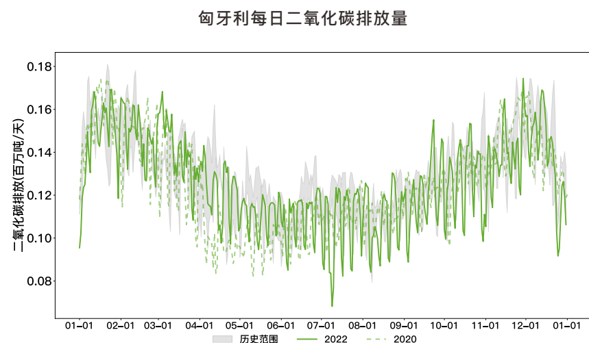
图3-74 2019年1月1日至2022年12月31日匈牙利每日二氧化碳排放量
