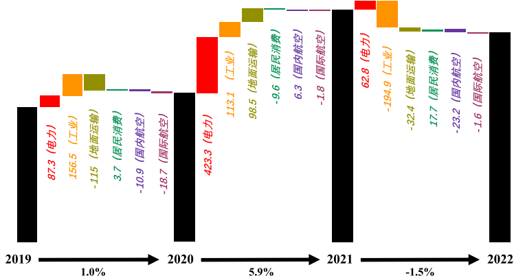
图3-86 2019-2022年 中国二氧化碳排放总量（黑色柱子）与各部门排放变化情况（彩色柱子）
