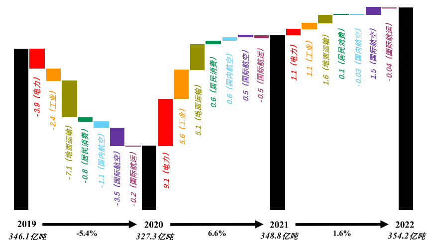
图2-3 2019-2022年二氧化碳排放总量（黑色柱子）与各部门排放变化情况（彩色柱子）
