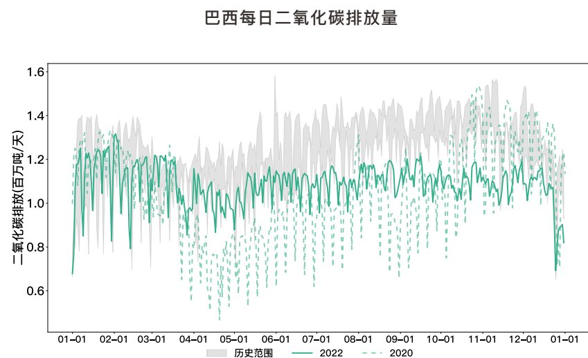
图3-92 2019年1月1日至2022年12月31日巴西二氧化碳排放日度变化情况
