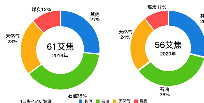
图3-6 欧盟27国&英国一次能源消费结构
