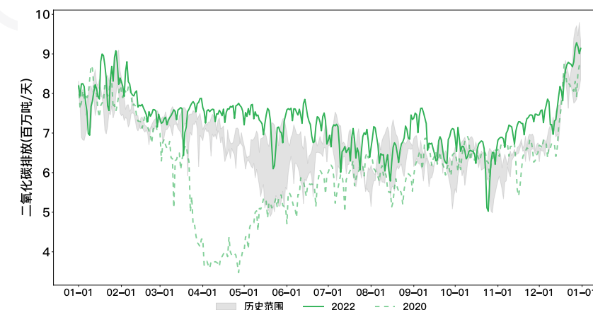
图3-88 2019年1月1日至2022年12月31日印度二氧化碳排放日度变化情况
