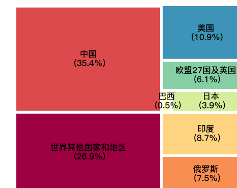
图2-5 2020年世界各国电力部门二氧化碳排放在全球电力部门二氧化碳总排放中占比
