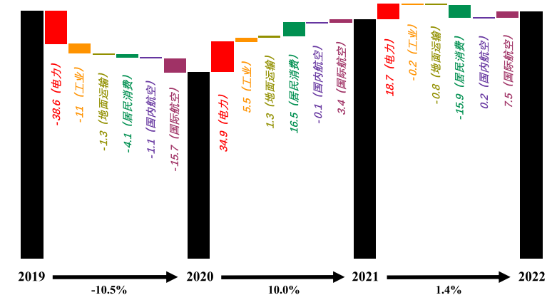
图3-16 2019-2022年德国二氧化碳排放总量（黑色柱子）与各部门排放变化情况（彩色柱子）
