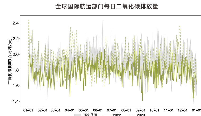
图2-16 2019年1月1日至2022年12月31日国际航运部门二氧化碳排放日度变化情况
