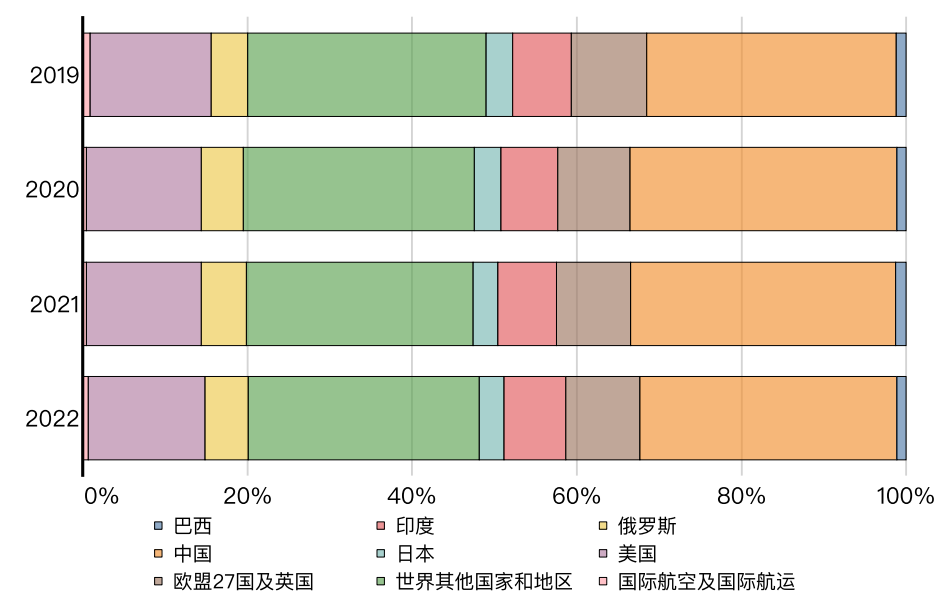
图2-2 2019–2022年各国二氧化碳排放占比
