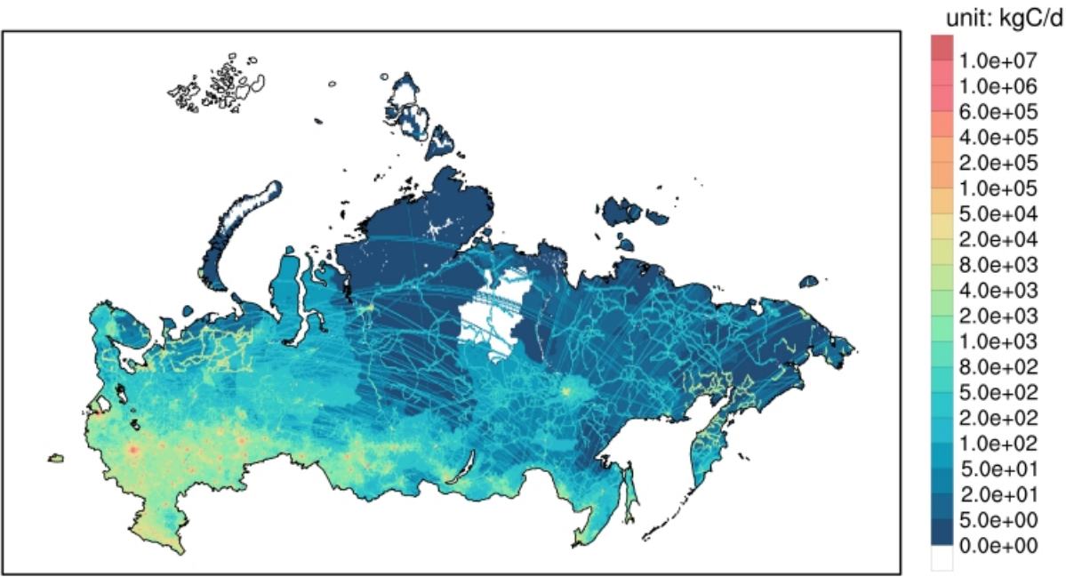
图3-83 2020年俄罗斯日均碳排放地图
