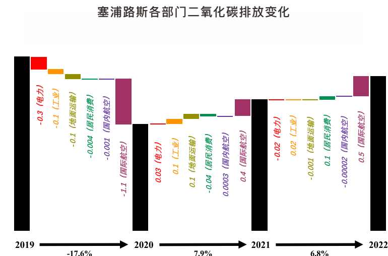
图3-67 2019-2022年塞浦路斯二氧化碳排放总量（黑色柱子）与各部门排放变化情况（彩色柱子）
