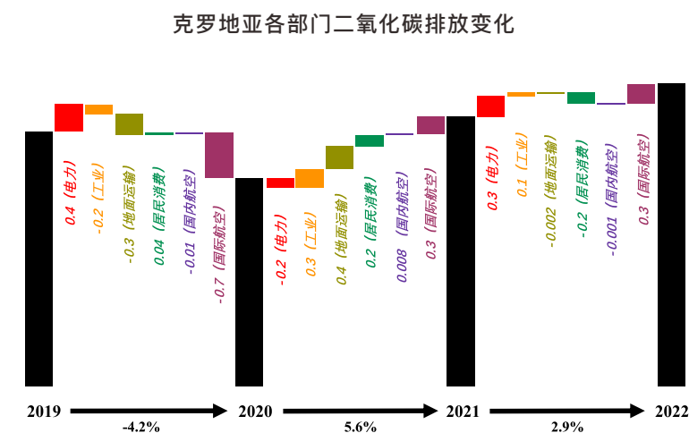
图3-51 2019-2022年克罗地亚二氧化碳排放总量（黑色柱子）与各部门排放变化情况（彩色柱子）
