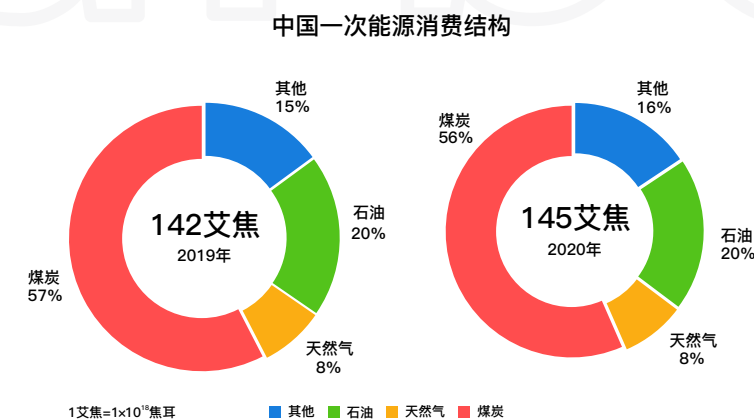
图3-84 中国一次能源消费结构
