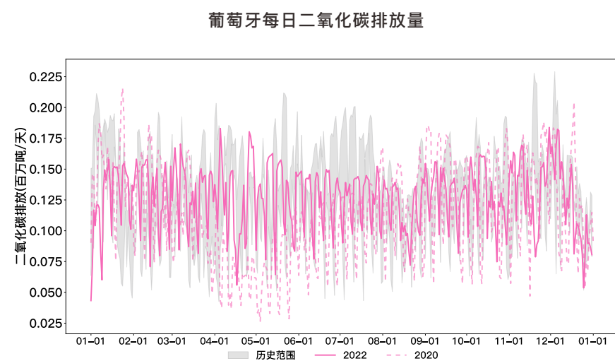
图3-62 2019年1月1日至2022年12月31日葡萄牙每日二氧化碳排放量
