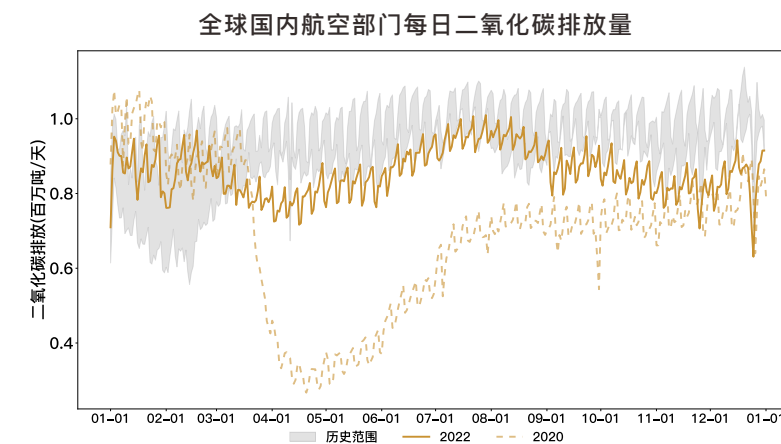
图2-12 2019年1月1日至2022年12月31日国内航空部门二氧化碳排放日度变化情况
