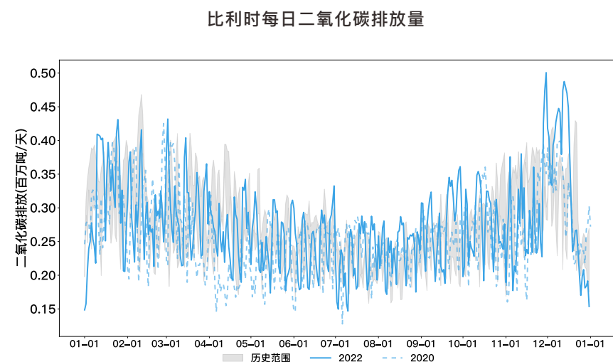
图3-38 2019年1月1日至2022年12月31日比利时每日二氧化碳排放量
