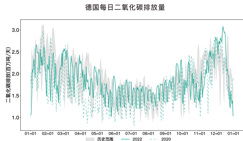
图3-15 2019年1月1日至2022年12月31日德国二氧化碳排放日度变化情况
