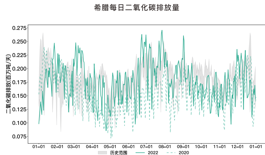
图3-72 2019年1月1日至2022年8月31日希腊每日二氧化碳排放量
